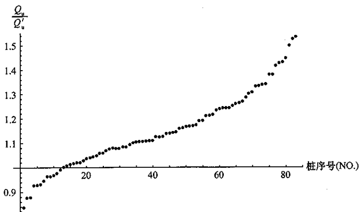
图 3 三岔双向挤扩灌注桩极限承载力实测值与式（2） 极限承载力估算值的比值
