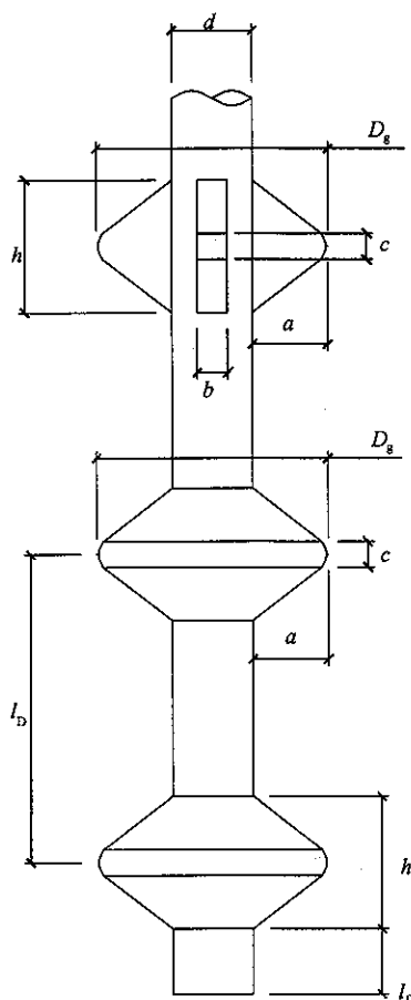
图 A 三岔双向挤扩灌注桩的构造示意 a —承力盘（岔）宽度； b —承力岔厚度； c —承力盘（岔）外沿高度； d —桩身设计直径； h —承力盘（岔）高度； D_g —承力盘（岔）公称直径； l_D —承力盘竖向间距； l_t —桩根长度
